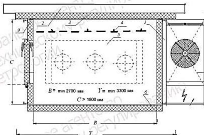
а) Внутренняя часть стенда (вид сверху)
