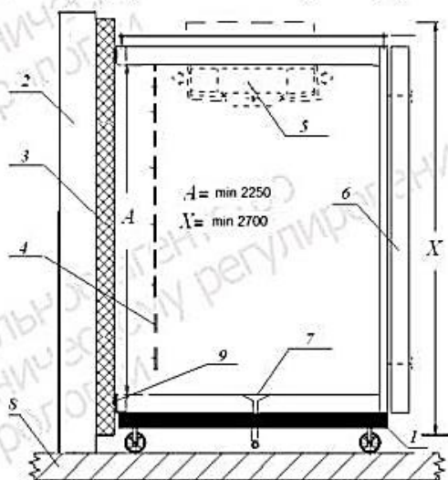
б) Внутренняя часть стенда (вид сбоку)
