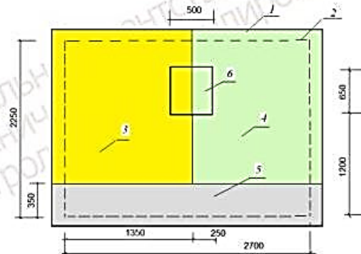
1 – фрагмент СФТК; 2 – участок, подвергаемый климатическим воздействиям; 3 – участок декоративно-защитного слоя 1-го вида; 4 – участок декоративно-защитного слоя 2-го вида (полный образец СФТК); 5 – участок базового армированного слоя (частичный образец СФТК); 6 – имитация оконного проема
